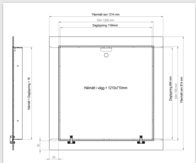
Exempel ritning: Underkantshängd lucka.
